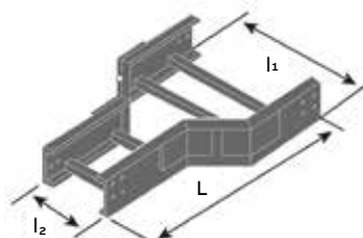
Réducteur rectiligne
