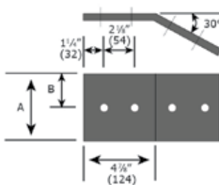
Éclisses 30° horizontales
