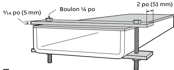
Bride de serrage de couvercle ultra-robuste
